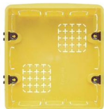
506E (108x118x51.5 mm)
